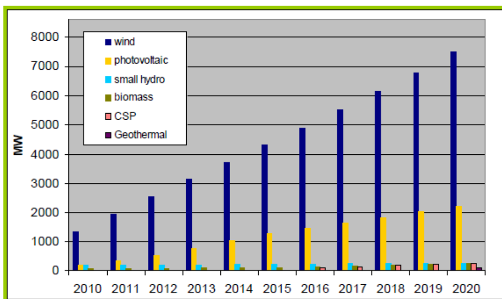
Σχήμα 29: Εκτιμώμενη εγκατεστημένη ισχύς από τις διάφορα είδη ΑΠΕ για το 2020
